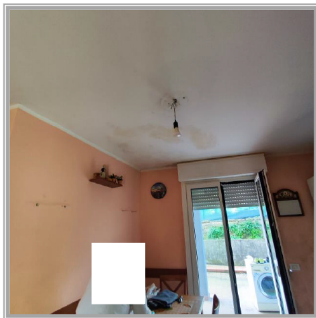
Fotografia 7 – Dettaglio umidità per condensa
