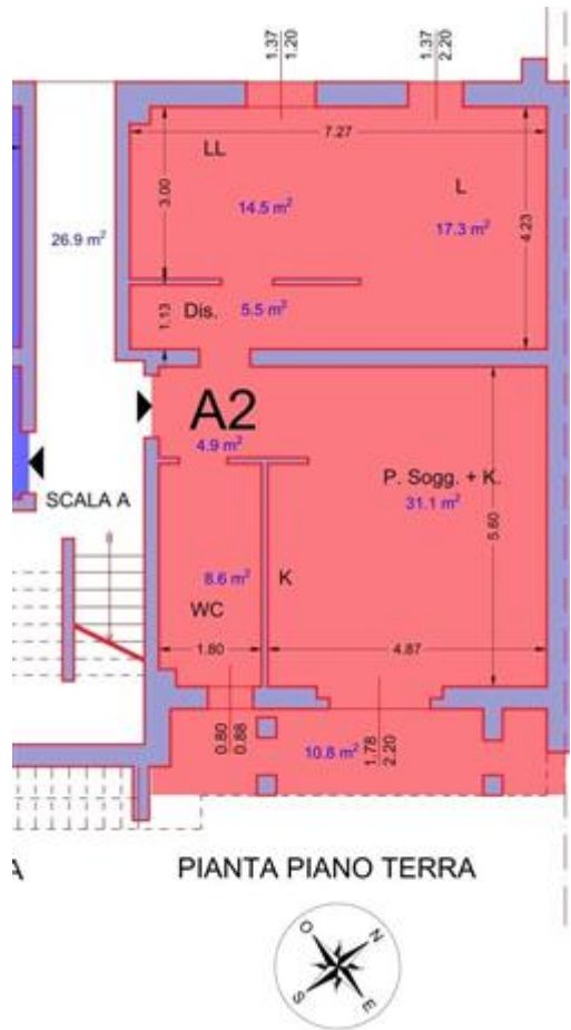
Pianta Appartamento A2
