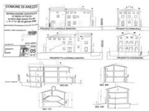
PROSPETTI E SEZIONI DELLO STATO AUTORIZZATO
