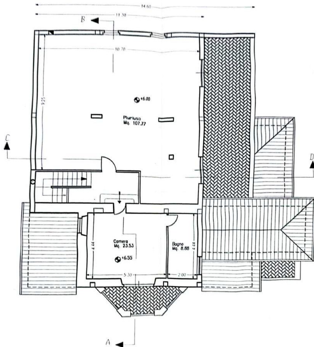
PIANTA PIANO SOTTOTETTO
