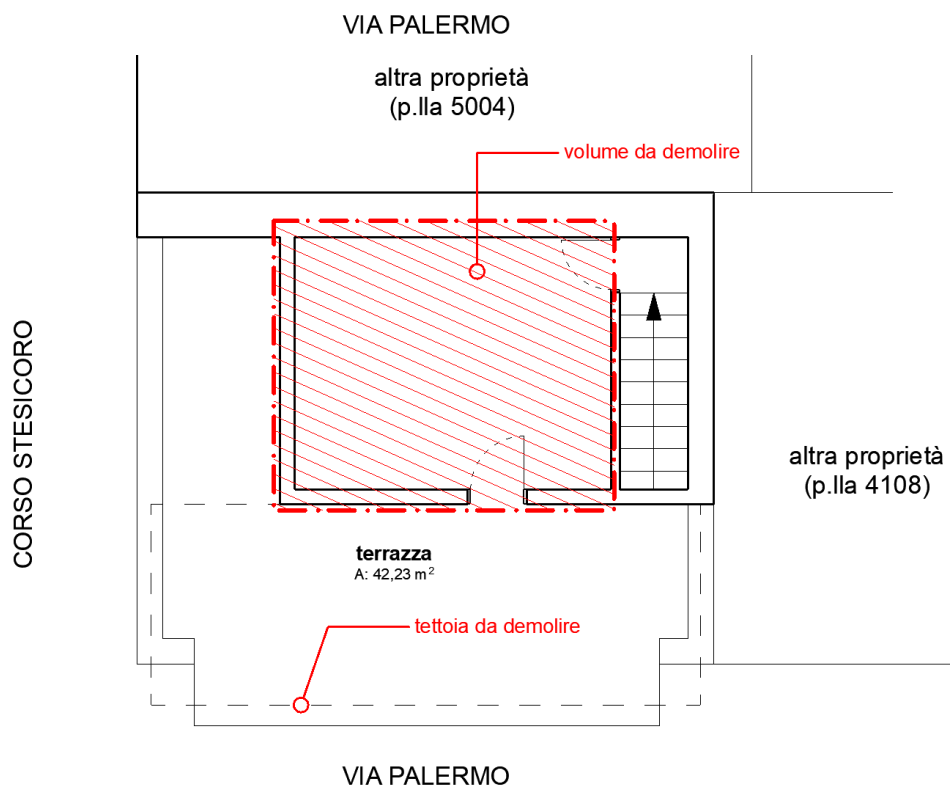
PIANTA COPERTURA
