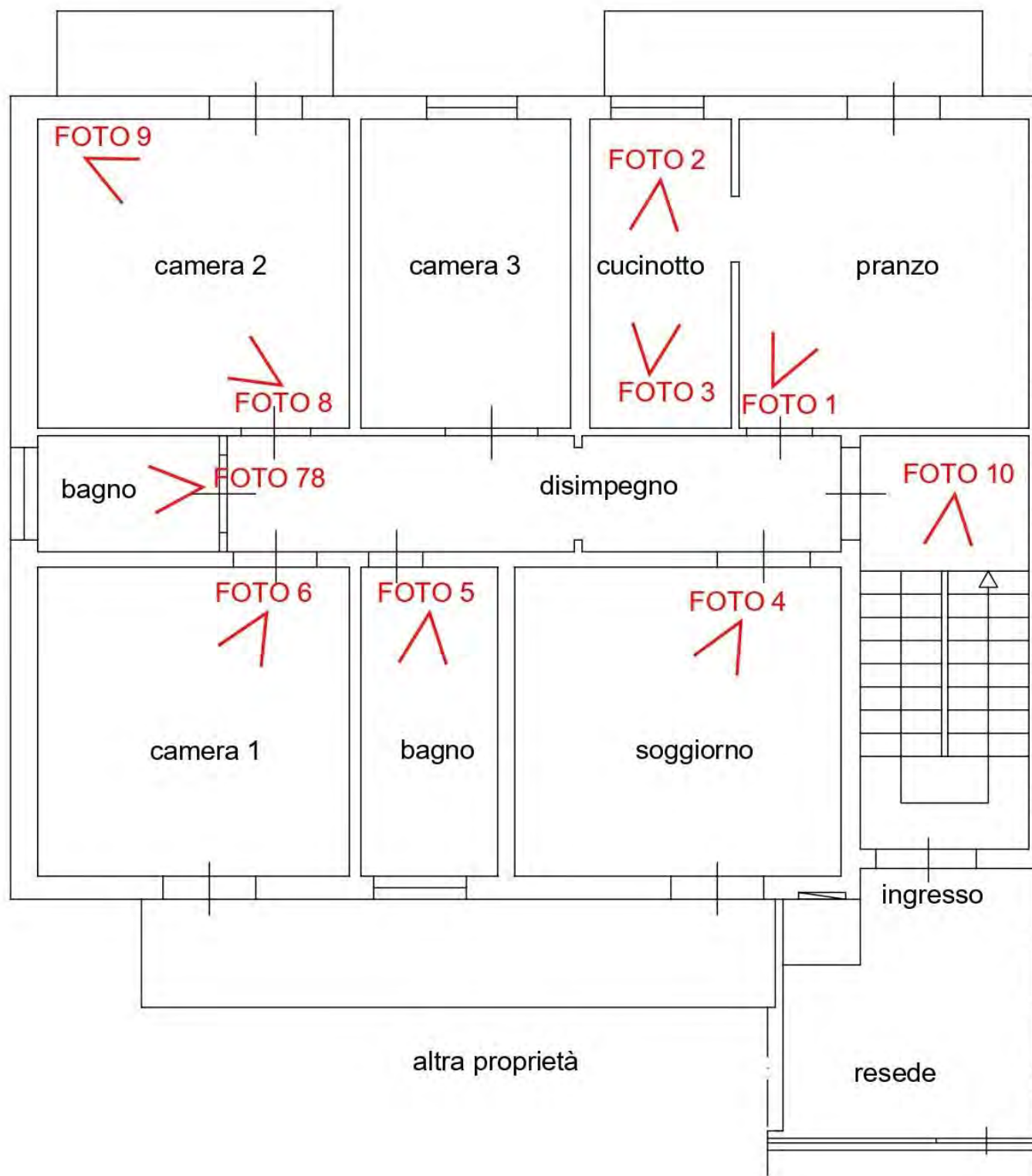
PIANTA PIANO PRIMO UNITA' "B"
